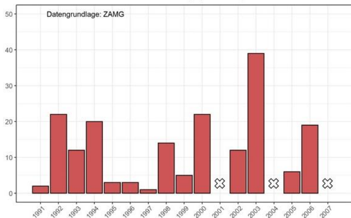
Anzahl der Hitzetage ( T_{\max} \geq 30^{\circ}\text{C} ) Station Wörterberg (1991-2007)
