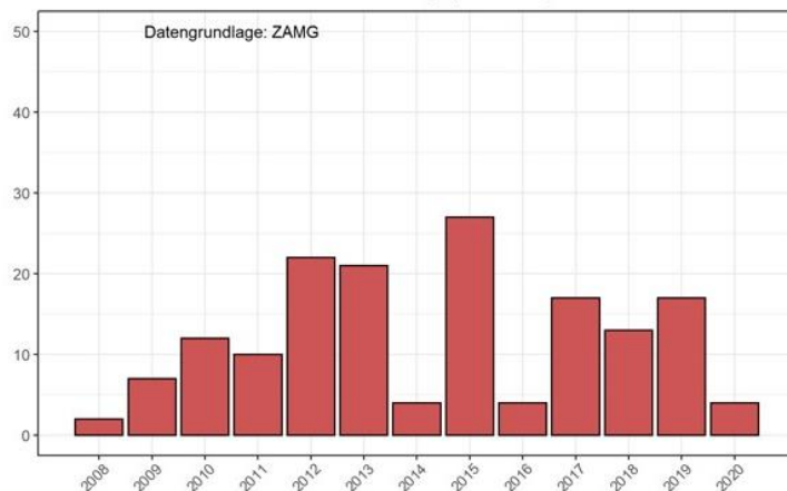
Anzahl der Hitzetage ( T_{\max} \geq 30^{\circ}\text{C} ) Station Wörterberg (2008-2020)
